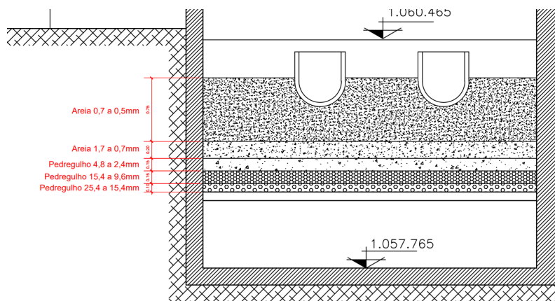
Figura 02 – Camadas de material filtrante.
