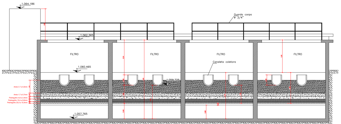
Figura 01 – Distribuição do material filtrante nos quatros filtros.
